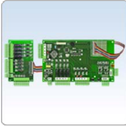
MINI PLC
